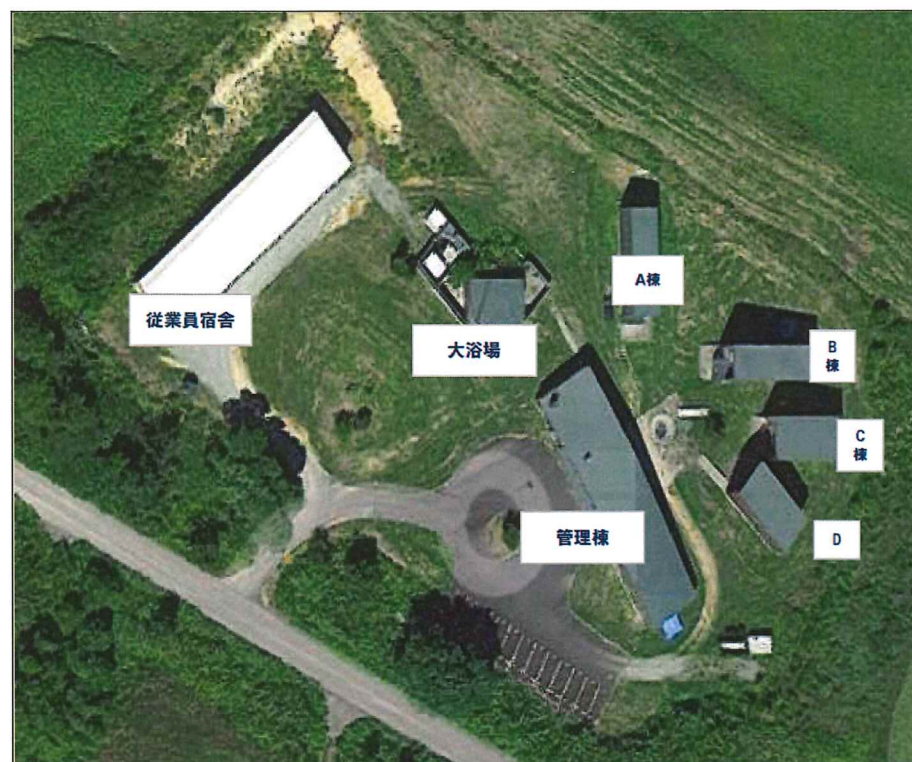
建物配置図
