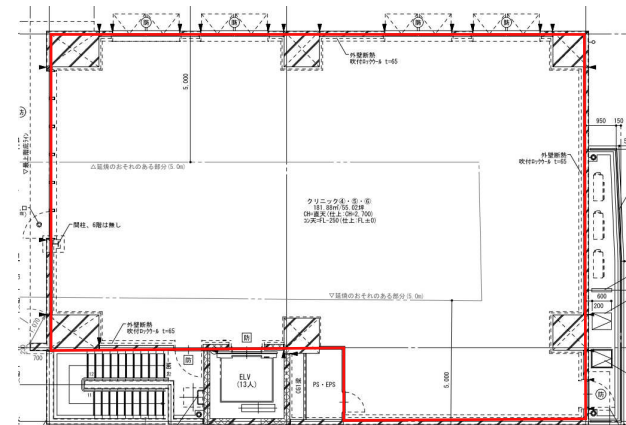
<4-6F 平面図>
