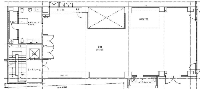
▲図面
